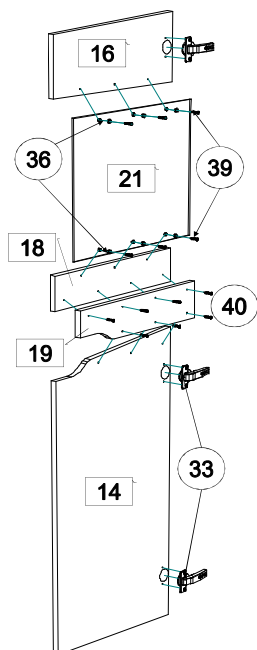
Эксцентриковая стяжка
